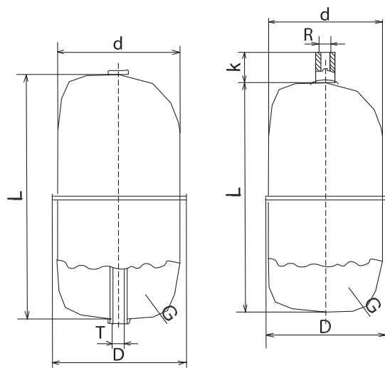
Резьбовое присоединение
